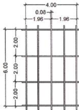
PLANTA
